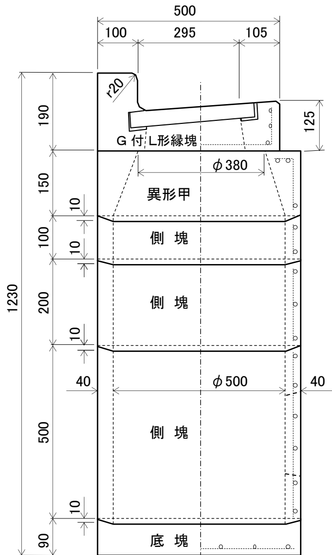
形状図
