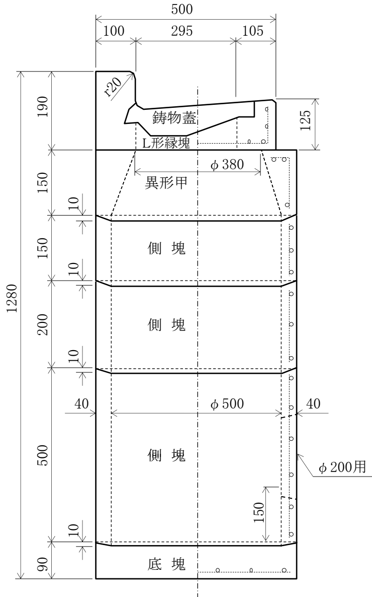
■ 形状図
