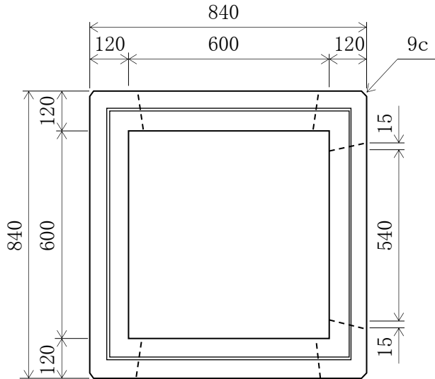
構造図
