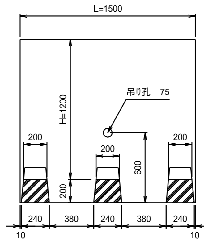
断面図
