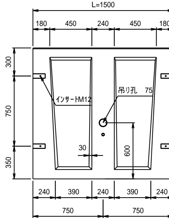
側面図
