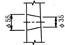
排水孔詳細図
