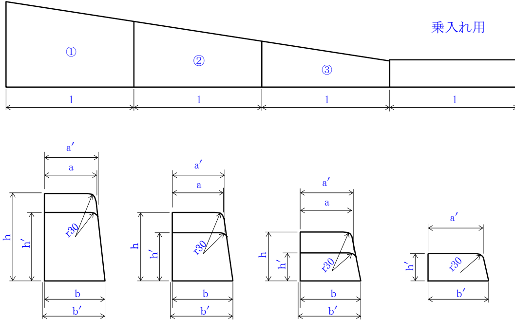
片面歩車道境界ブロック3段下り
