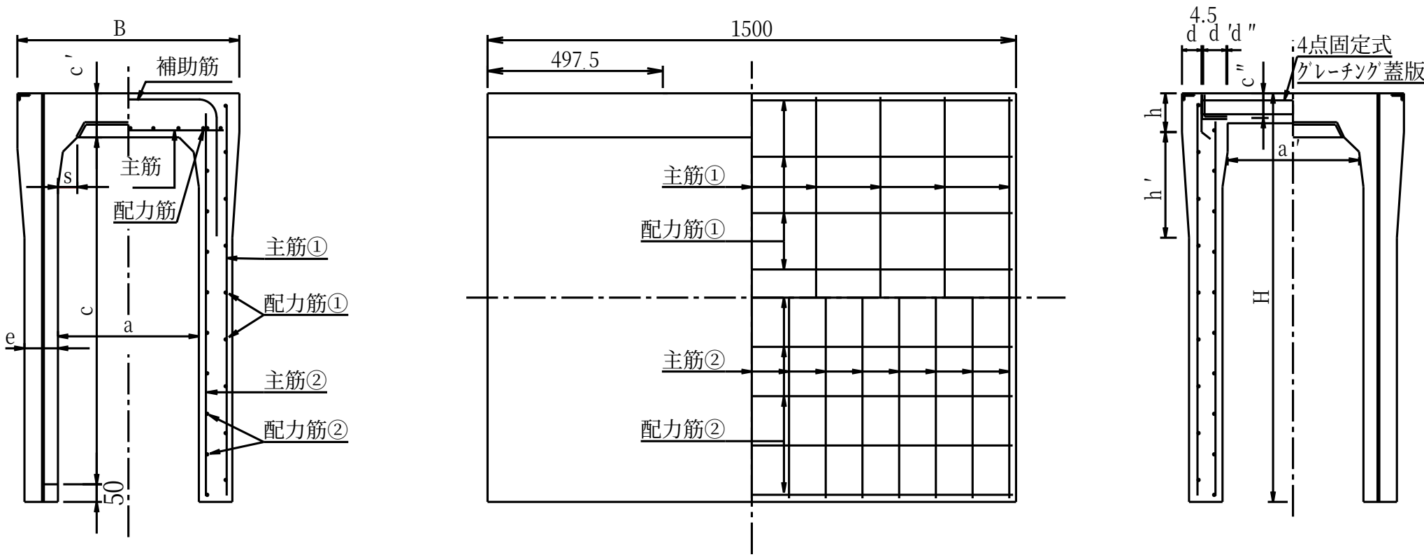
■寸法・配筋・重量
