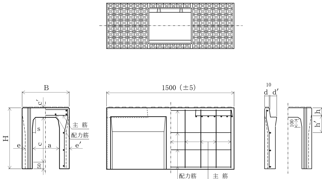
■ 形状図 (水路幅600)
