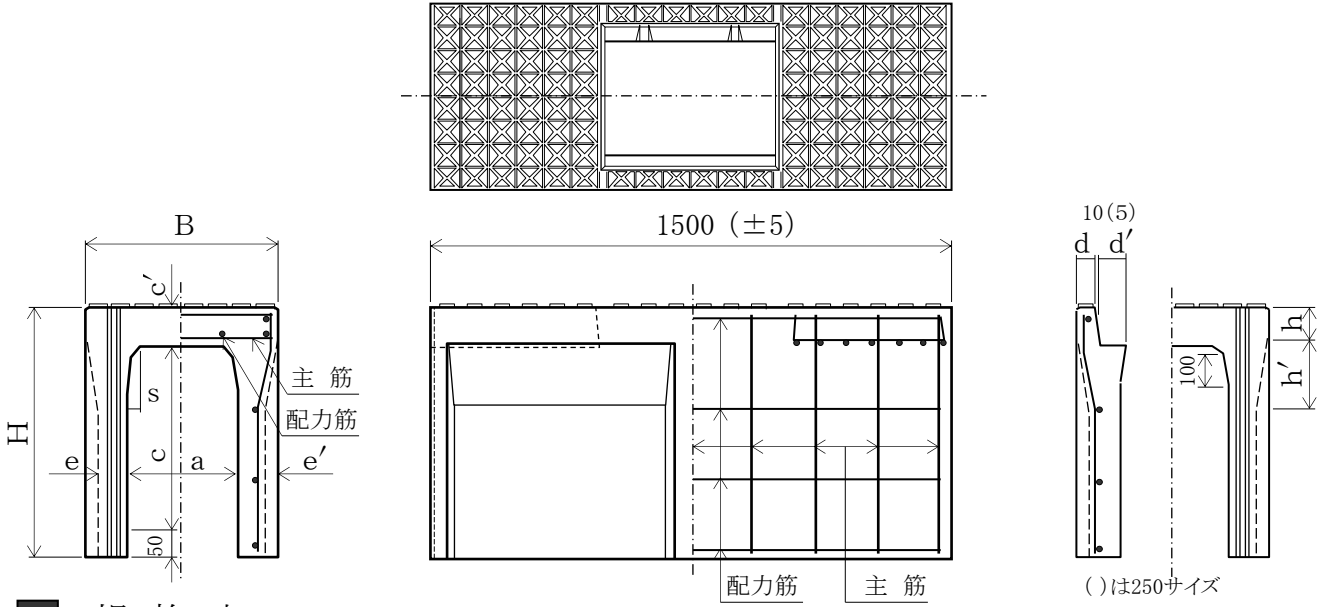
■ 規格表
