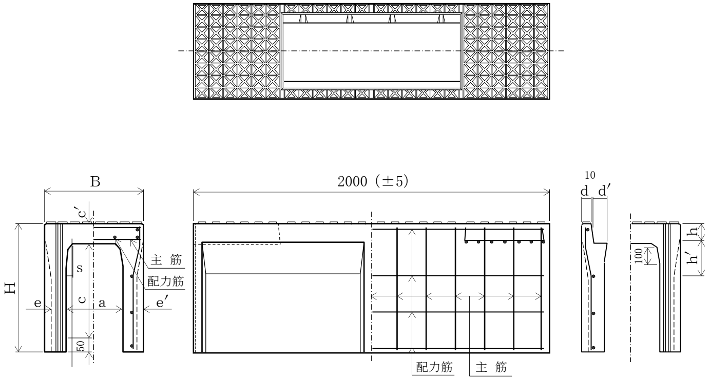
■ 形状図 (水路幅600)
