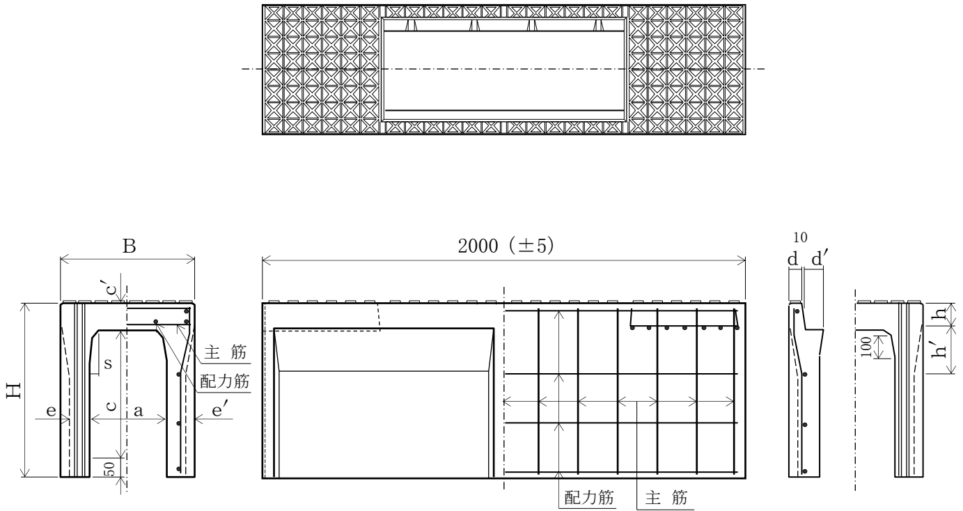
■ 形状図 (水路幅500)
