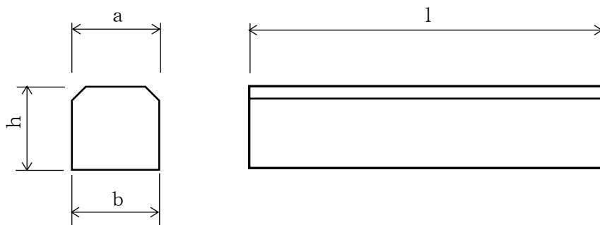
地先境界ブロック 面取り付
