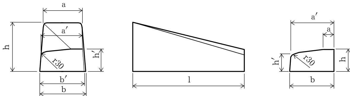
両面歩車道境界ブロック片下り
