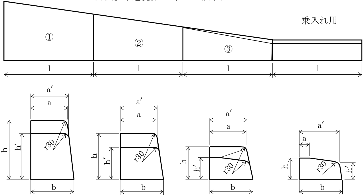
片面歩車道境界ブロックC3段下り
