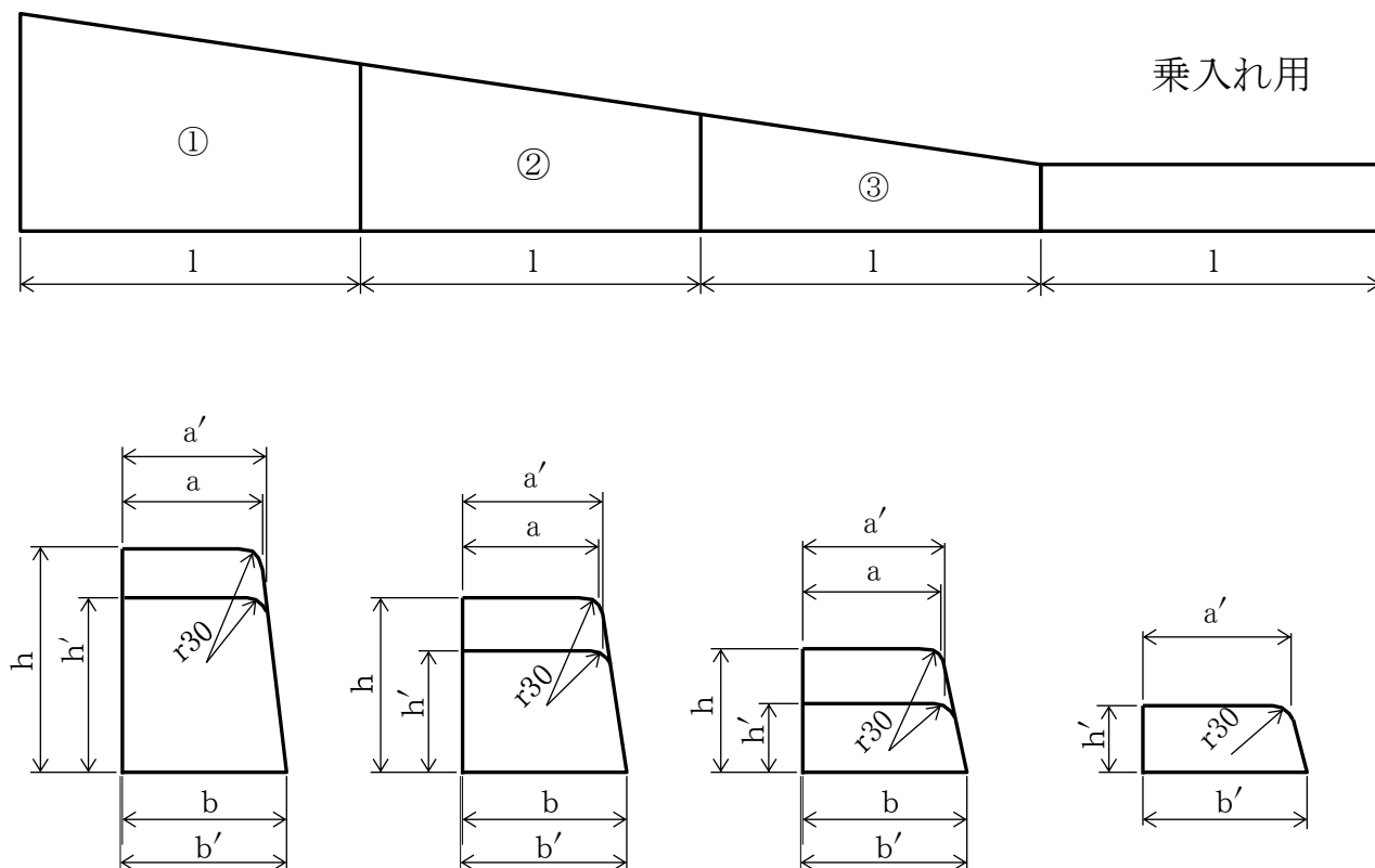
片面歩車道境界ブロック3段下り
