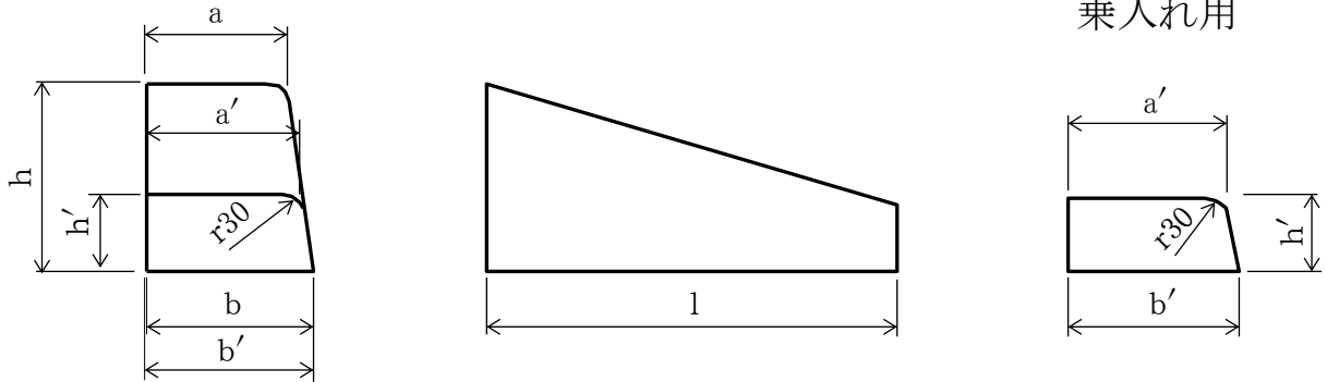
片面歩車道境界ブロック片下り
