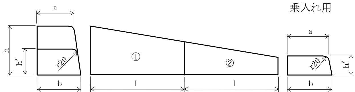
片面歩車道境界ブロック2段下り
