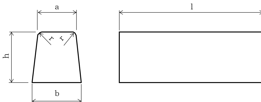
両面歩車道境界ブロック
