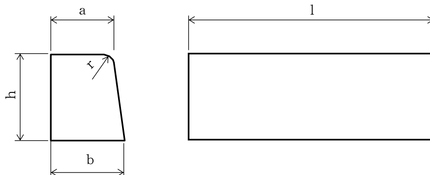
片面歩車道境界ブロック
